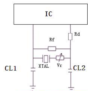
Negative impedance test diagram 负性阻抗测试示意图
