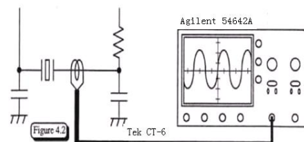
Drive level 测量示意图
